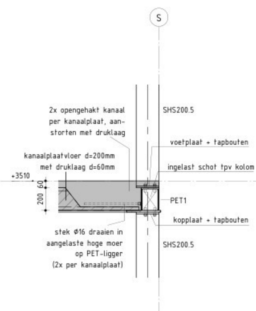
Detail 12 SCHAAL 1 : 20
