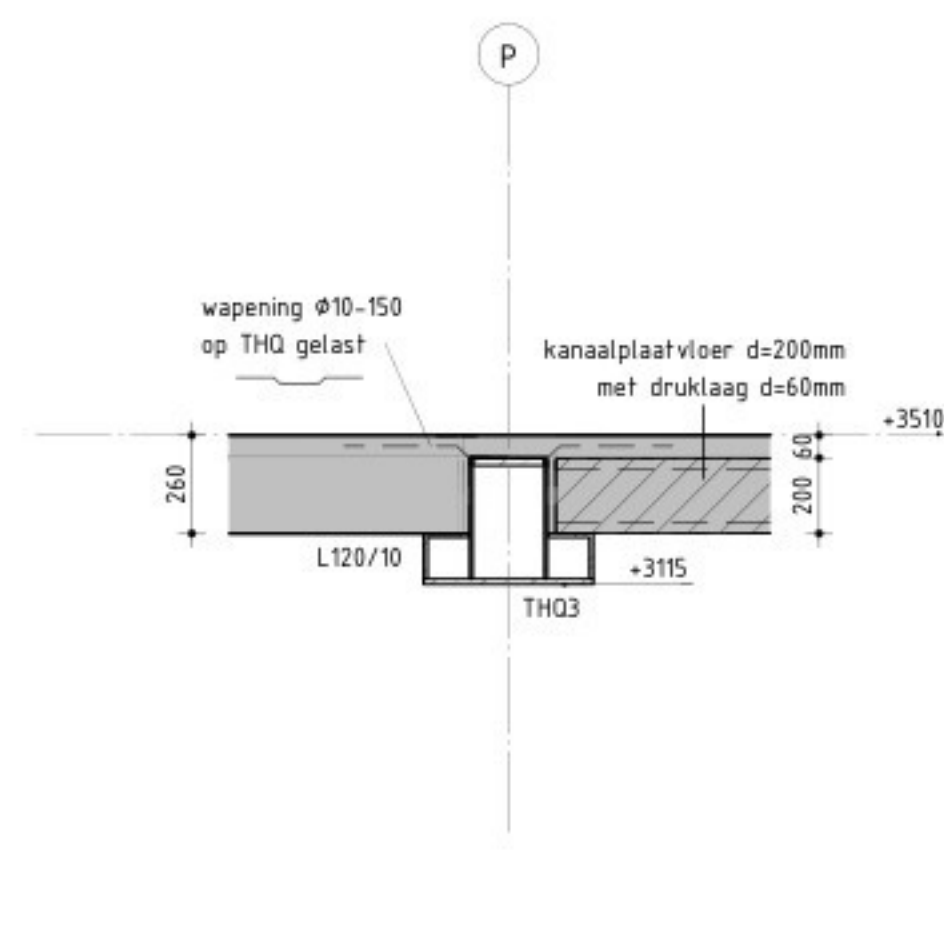
Detail 1.12 SCHAAL 1 : 20
