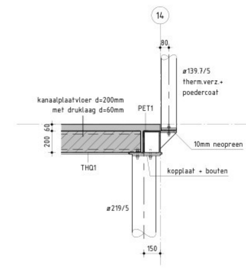
Detail 1.13 SCHAAL 1 : 20
