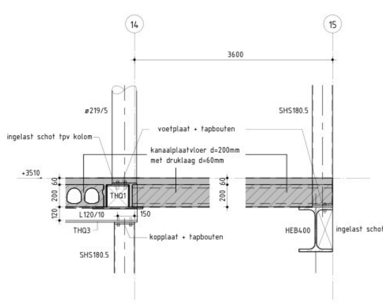
Detail 15 SCHAAL 1 : 20
