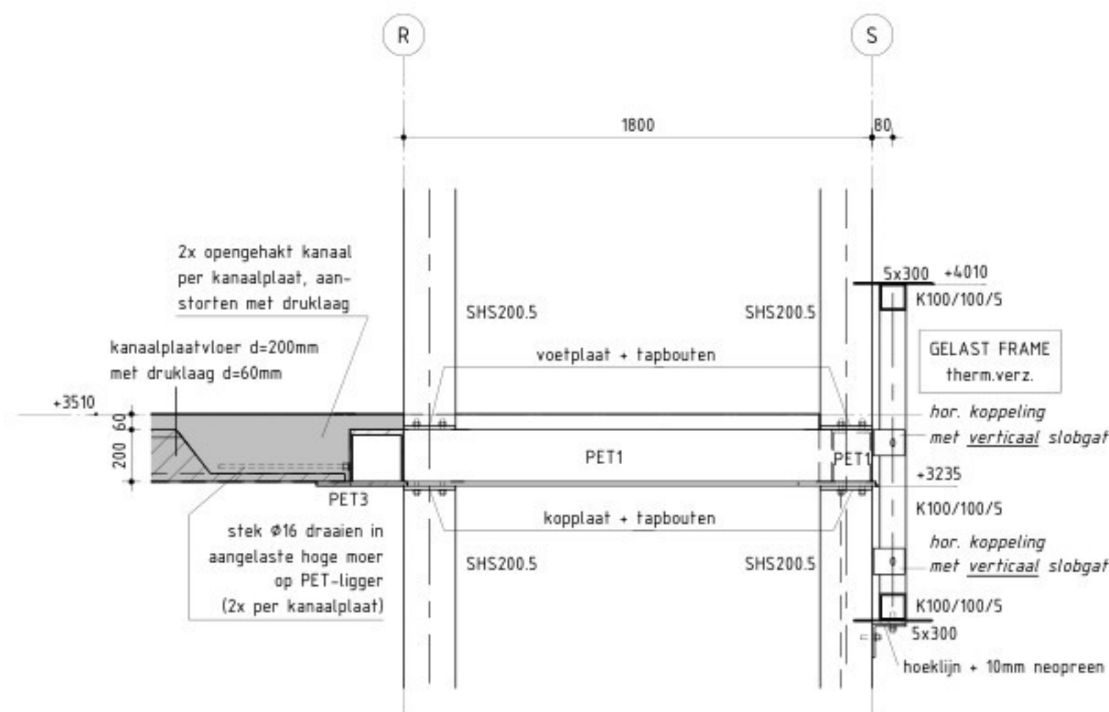
Detail 11 SCHAAL 1 : 20
