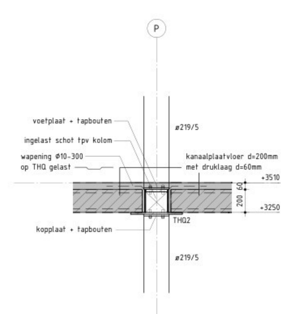
Detail 14 SCHAAL 1 : 20
