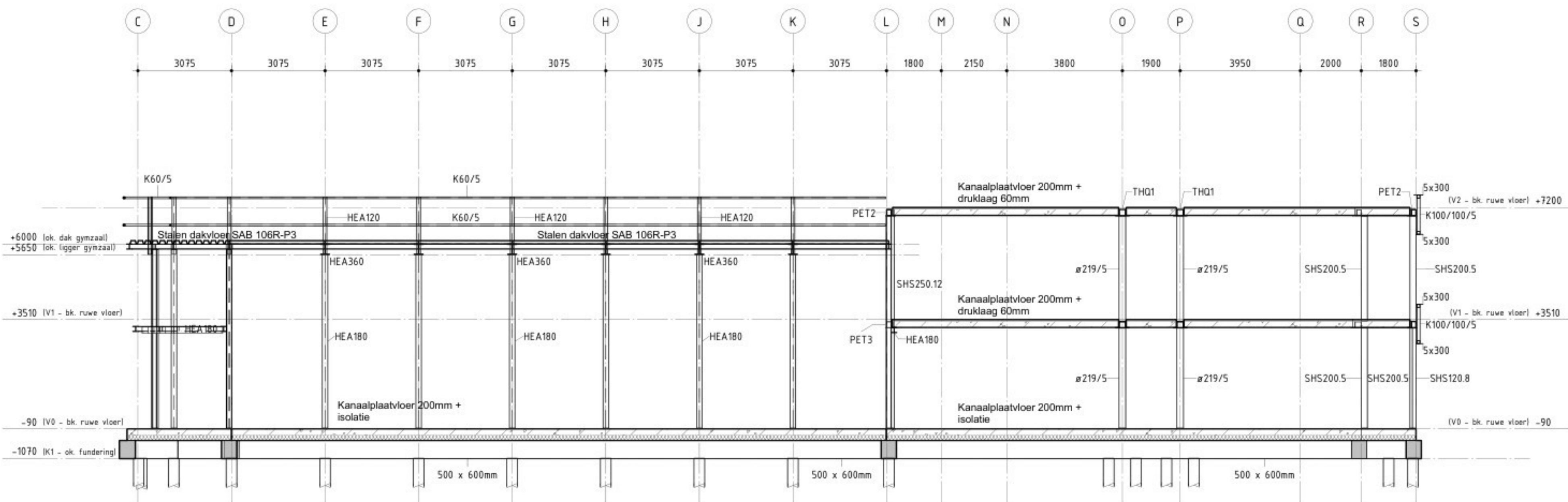
DWARSDOORSNEDE B-B SCHAAL 1 : 100
