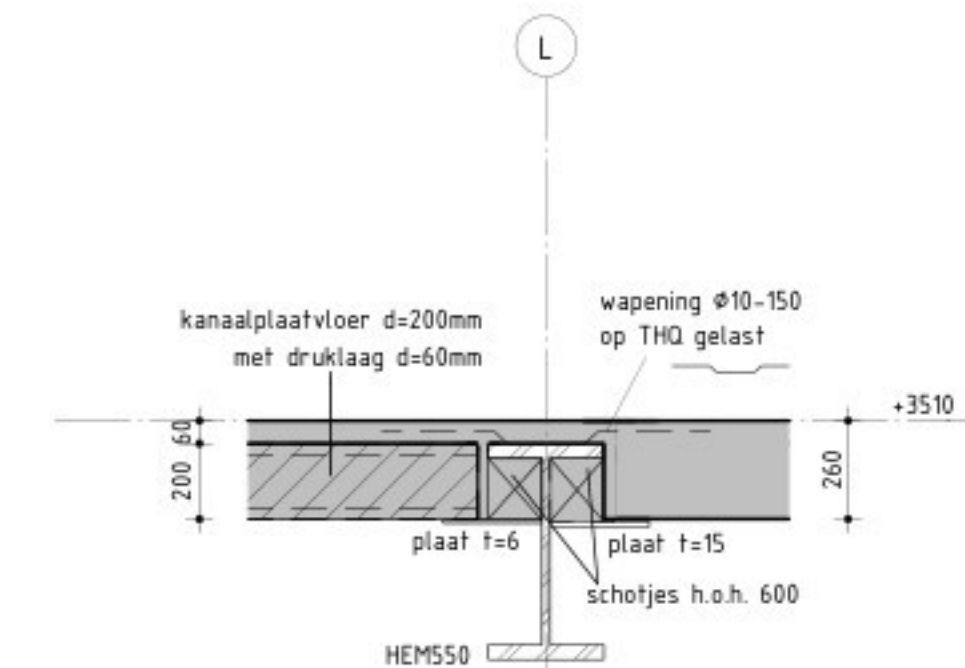
Detail 19 SCHAAL 1 : 20
