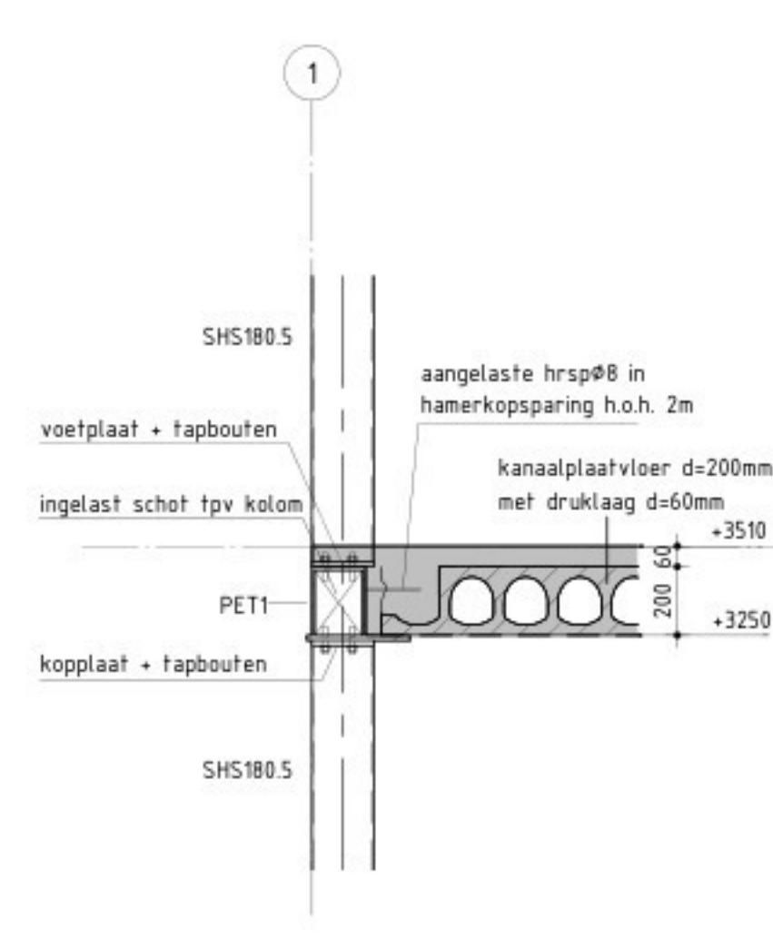
Detail 13 SCHAAL 1 : 20
