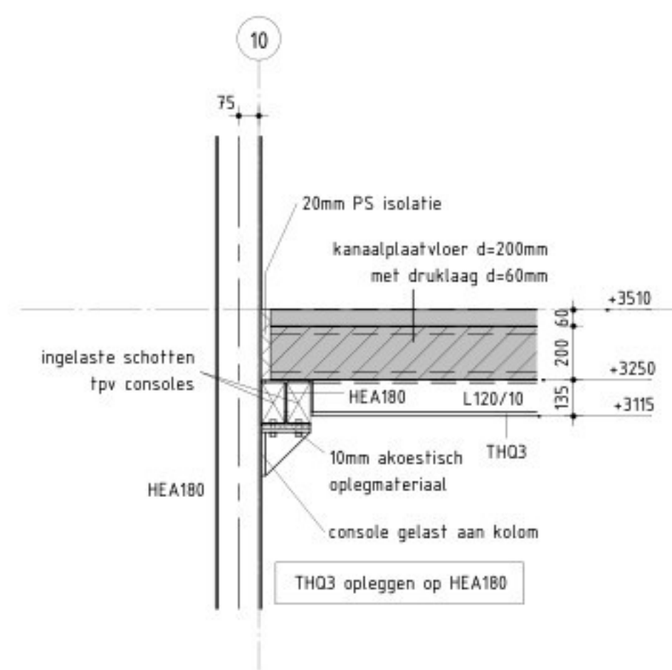
Detail 1.10 SCHAAL 1 : 20
