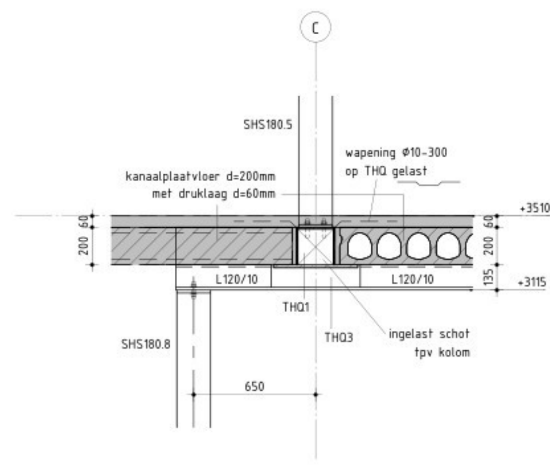
Detail 1.11 SCHAAL 1 : 20
