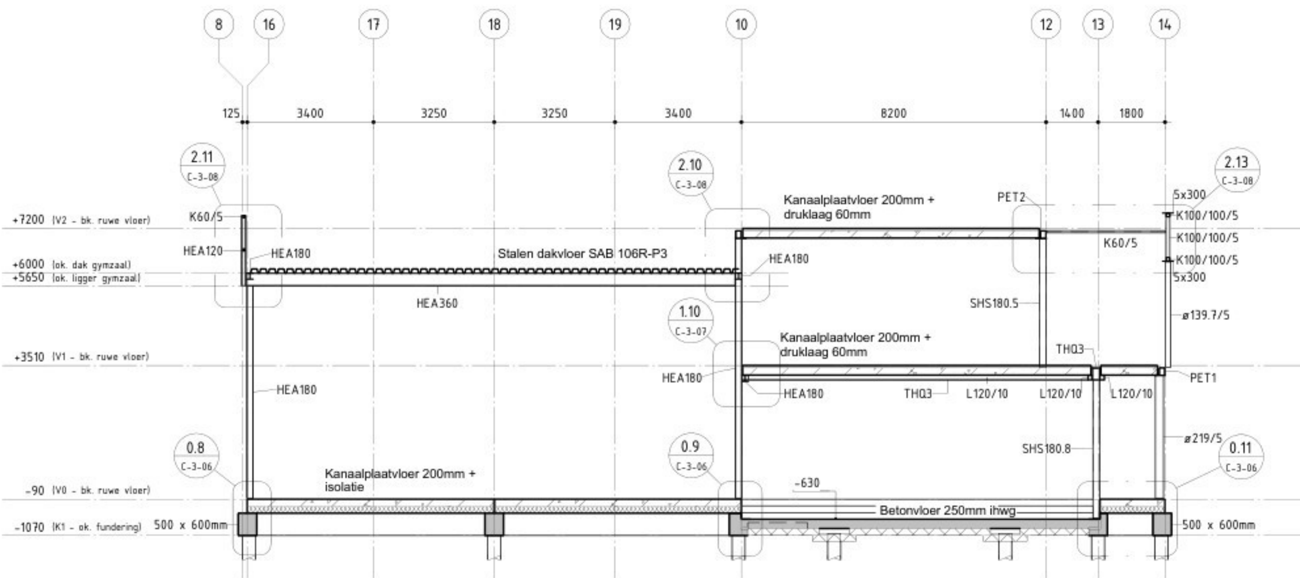
DWARSDOORSNEDE A-A SCHAAL 1 : 100
